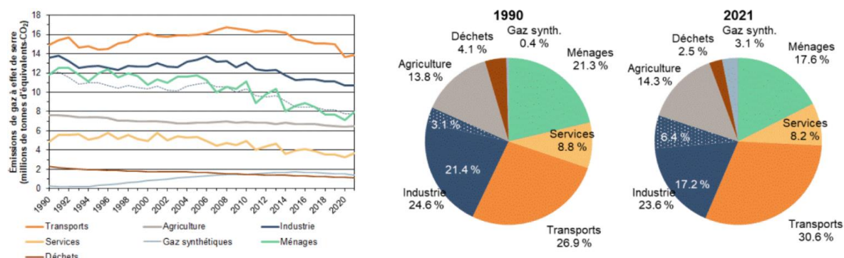
Figure 1 : graphique de gauche : évolution des émissions de GES entre 1990 et 2021 par secteur, en millions de t d'éq.-CO 2 / graphique de droite : part des secteurs dans le total des émissions de GES en 1990 et 2021 (secteur « bâtiment » = ménages et services ; zone en pointillés = émissions dues à l'incinération des déchets et à l'utilisation des déchets comme combustibles de substitution) 5
