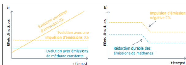
Fig. 4 : comparaison de l'impact climatique de l'évolution des émissions de CO 2 et de méthane en cas d'émissions constantes (a) et de réduction des émissions (b) 13
