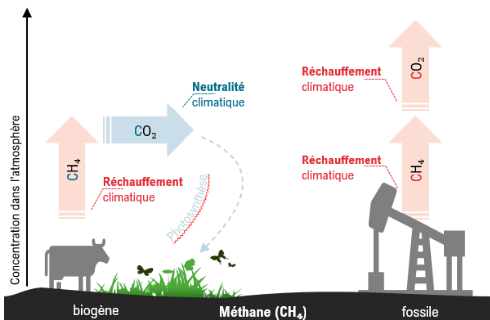
Fig. 5 : effets du méthane biogène et du méthane fossile sur le climat 16
