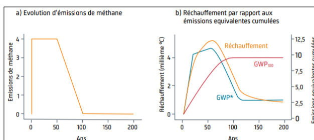
Fig. 6 : le PRP* reflète mieux les évolutions temporelles et donc l'impact climatique des gaz continus à courte durée de vie que le PRP 100 13 .
