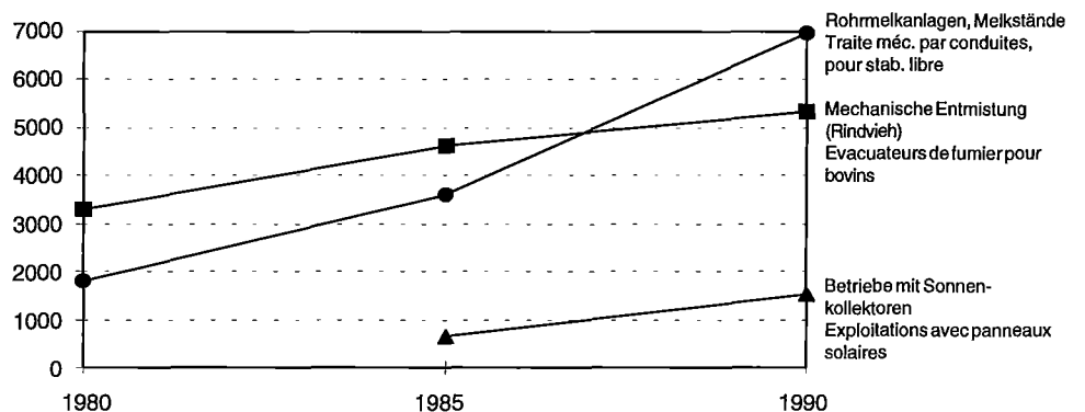
Zahlenmässige Entwicklung von Einrichtungen auf Produktionsbetrieben Evolution en chiffres des installations dans les exploitations de production
